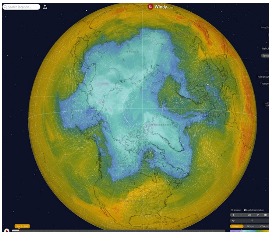
Rysunek 12: Rozkład temperatur na poziomie 850 hPa. Projekcja mapy od strony bieguna północnego. Należy zauważyć „języki” zimnego powietrza rozpełzające się od bieguna i języki ciepłego powietrza sunące w kierunku bieguna.
