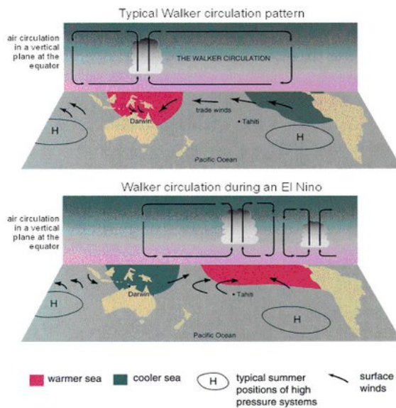
Rysunek 9: Typowa cyrkulacja Walkera (górny rysunek) oraz cyrkulacja w czasie El Nino: kolor różowy – cieplejsza woda, zielonkawy – chłodniejsza.
